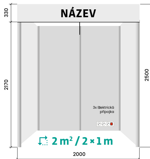
čelní pohled
